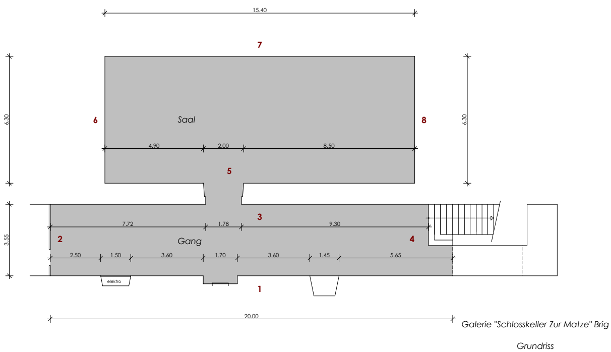
Grundriss
